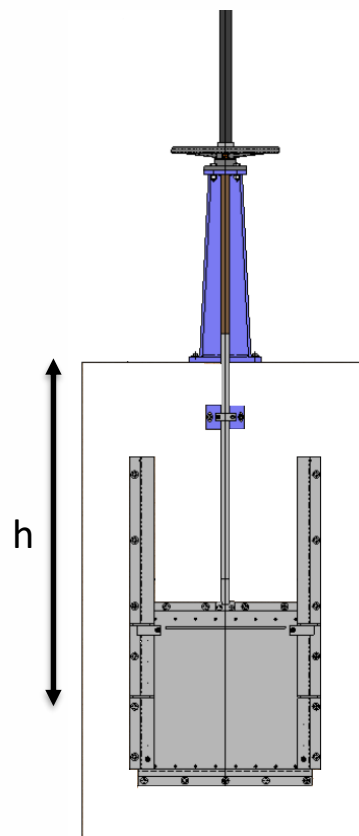
Pedestal de suspensão com engrenagens de redução simples e indicador de posição
